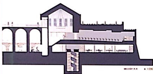
sezioni A-A 1/250
