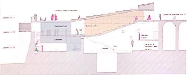
Sección longitudinal E 1/200
