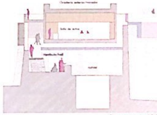
Sección transversal E 1/200
